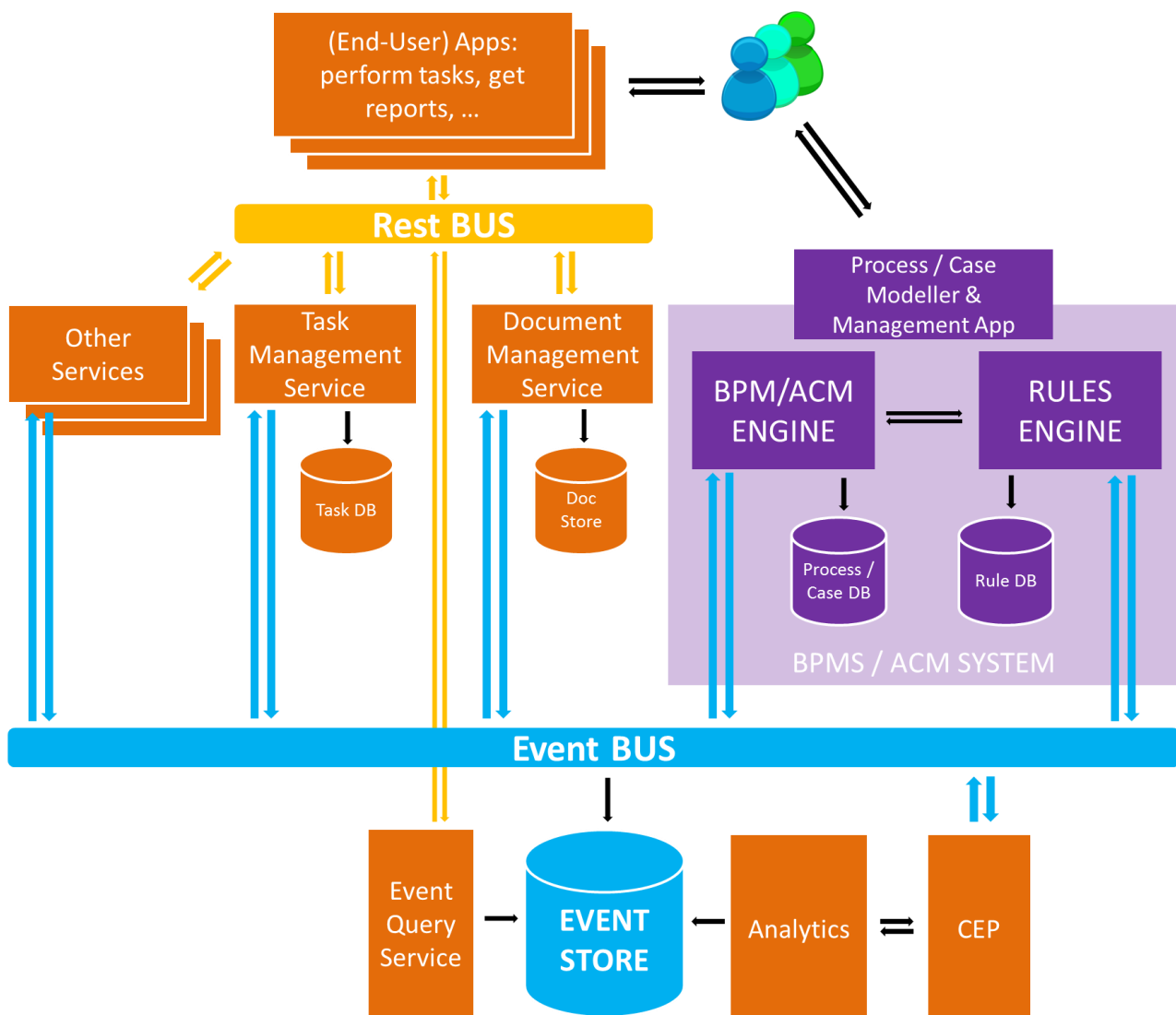
Fig. 9: Een voorbeeld van een modulaar stelsel van applicaties en diensten waarbinnen process en case management een centrale en orchestrerende rol spelen. De paarse delen maken typisch deel uit van een BPMS / ACM-systeem, maar ook een aantal van de andere (oranje) zaken zijn vaak in dergelijke suites opgenomen.
