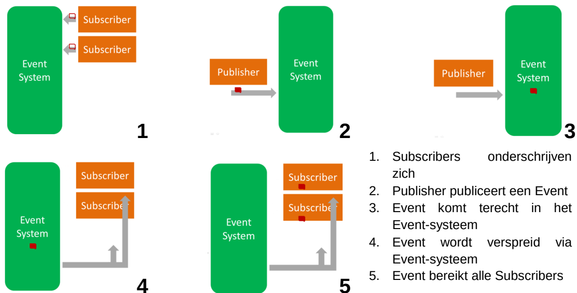
Fig. 4: Het publish / subscribe scenario, gebruik makende van Events
